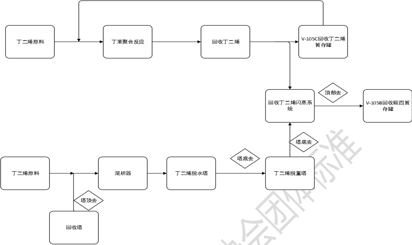
图 1 碳四回收料回收流程示意图
