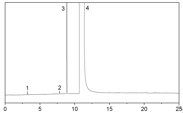
1-乙烷 2-反-2-丁烯 3-顺-2-丁烯 4-1,3-丁二烯 图 3 工业用丁二烯实际样品的典型色谱图
